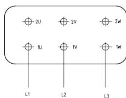
niedrige Drehzahl
