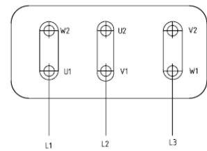
niedrige Spannung
