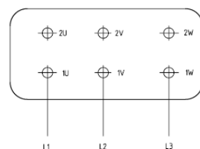
niedrige Drehzahl
